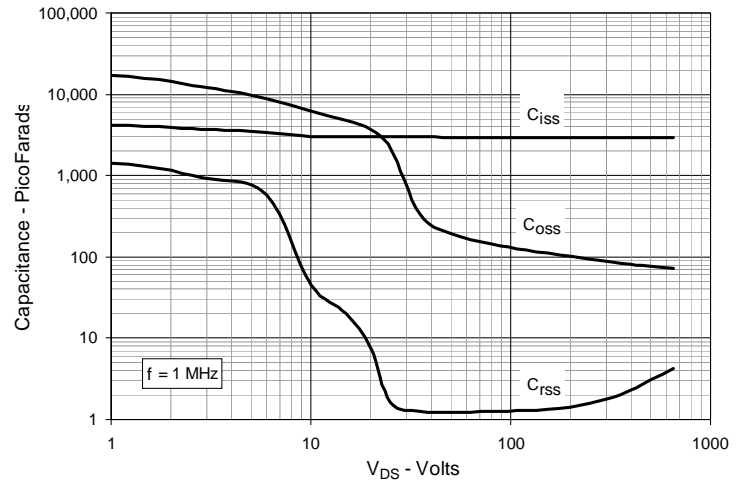
Fig. 12. Capacitance
